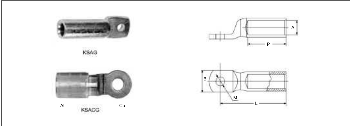
KSAG Końcówka szczelna dla żył Al wg normy DIN 46329
